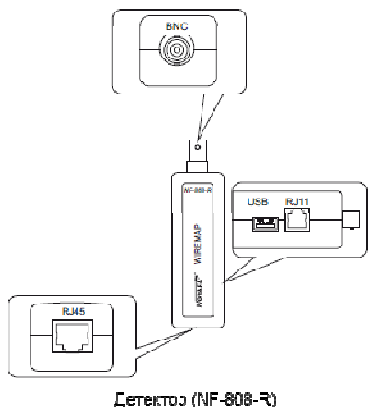
Детектор (NF-868-R)
