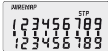
для экранированного кабеля RJ45
