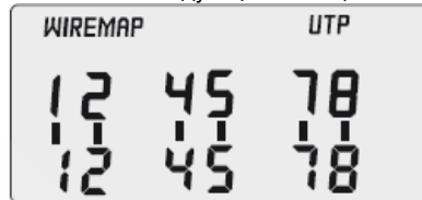
Результат при обрыве линий «3» и «6» кабеля RJ45
